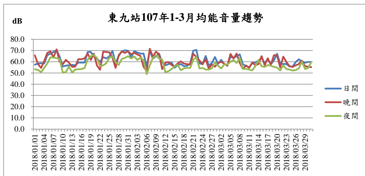
圖9 基隆港東九站107年1-3月噪音監測結果趨勢圖
