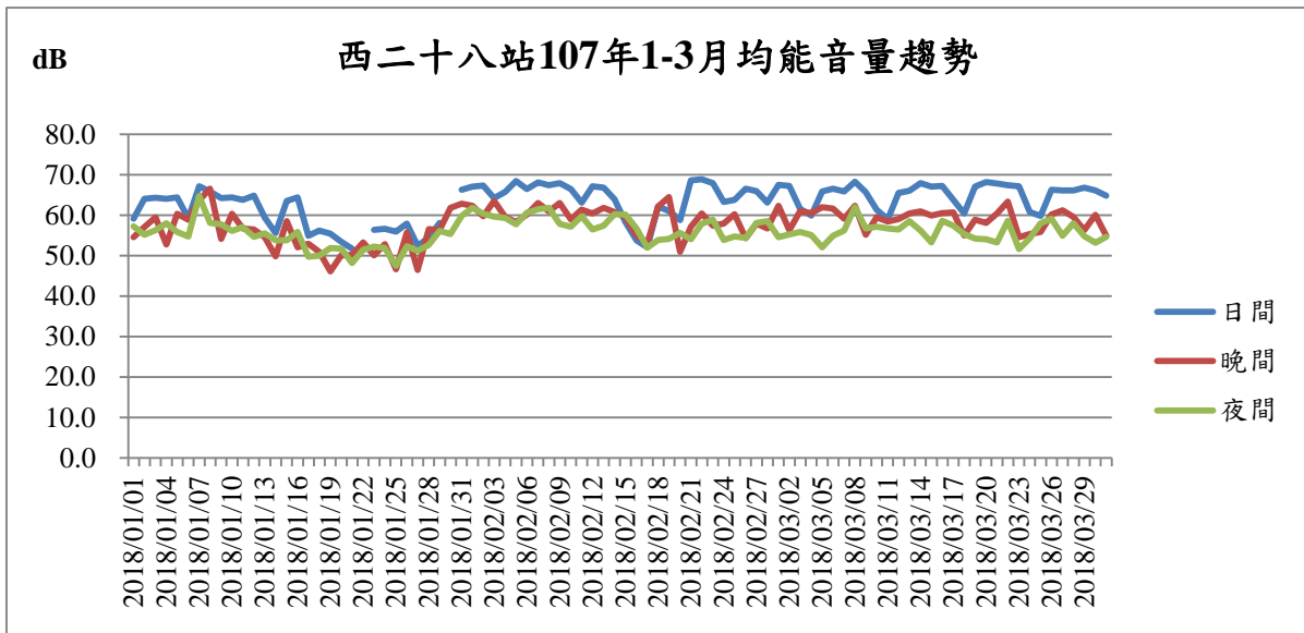
圖10 基隆港西二十八站107年1-3月噪音監測結果趨勢圖
