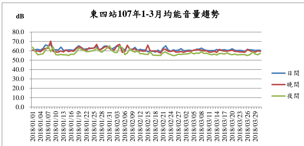
圖8 基隆港東四站107年1-3月噪音監測結果趨勢圖
