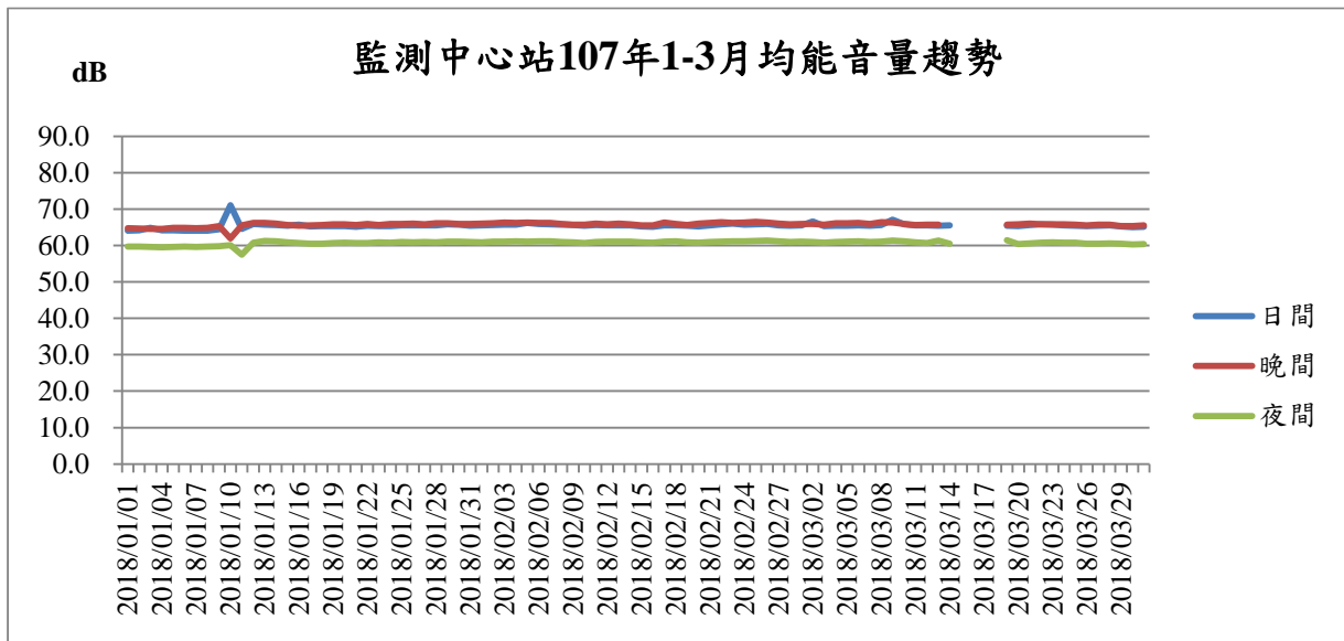
圖6 基隆港監測中心站107年1-3月噪音監測結果趨勢圖
