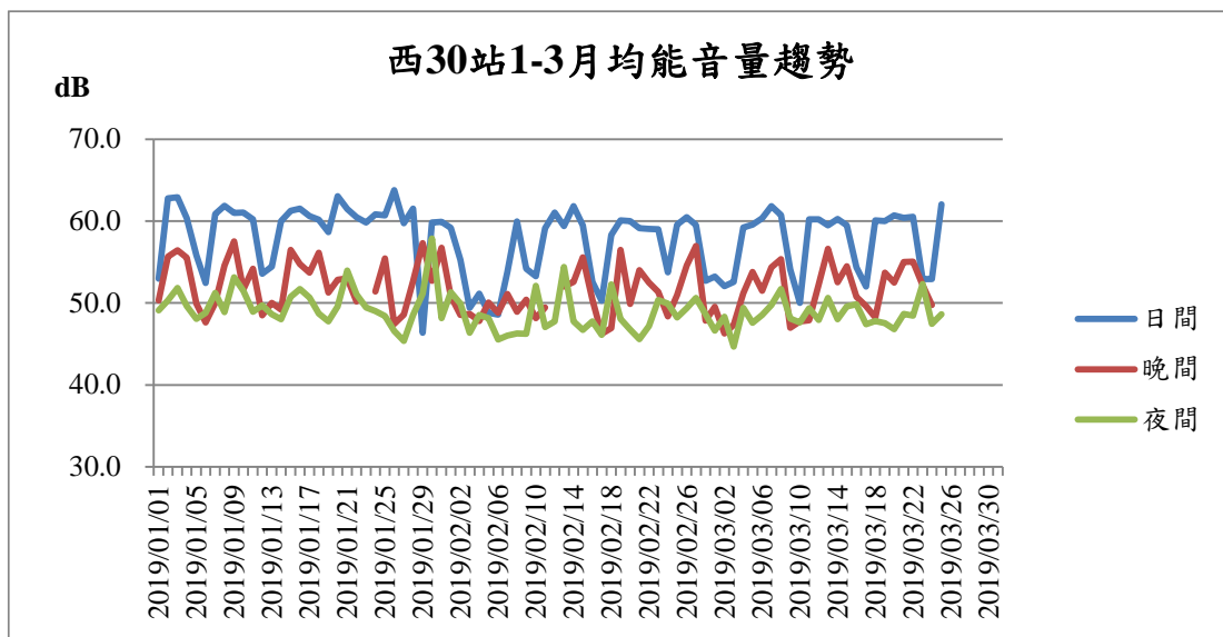
圖11 基隆港西三十站108年1-3月噪音監測結果趨勢圖
