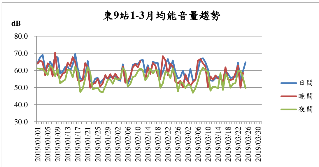
圖9 基隆港東九站108年1-3月噪音監測結果趨勢圖
