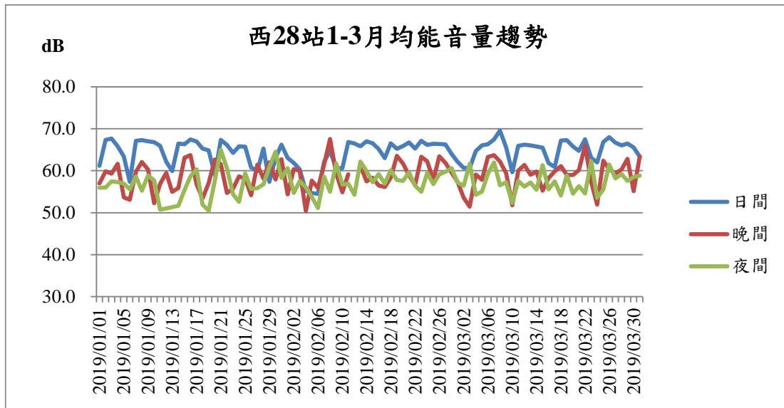
圖10 基隆港西二十八站108年1-3月噪音監測結果趨勢圖
