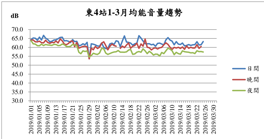
圖8 基隆港東四站108年1-3月噪音監測結果趨勢圖
