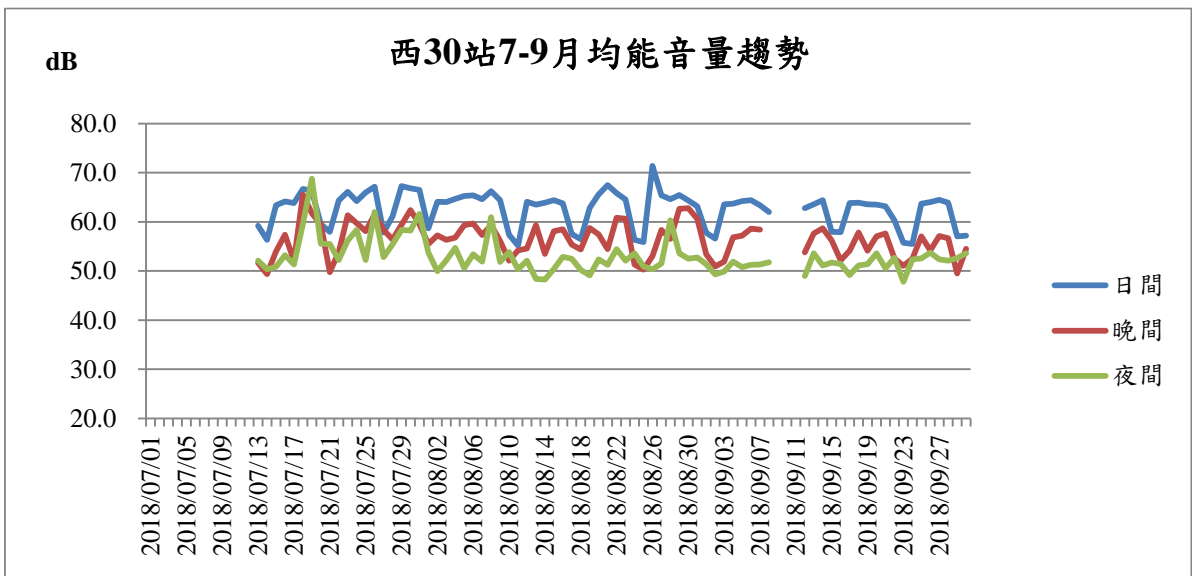
圖11 基隆港西三十站107年7-9月噪音監測結果趨勢圖
