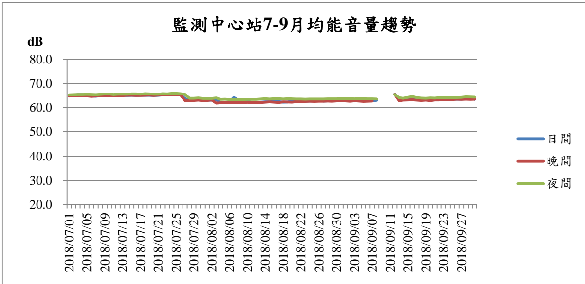
圖6 基隆港監測中心站107年7-9月噪音監測結果趨勢圖
