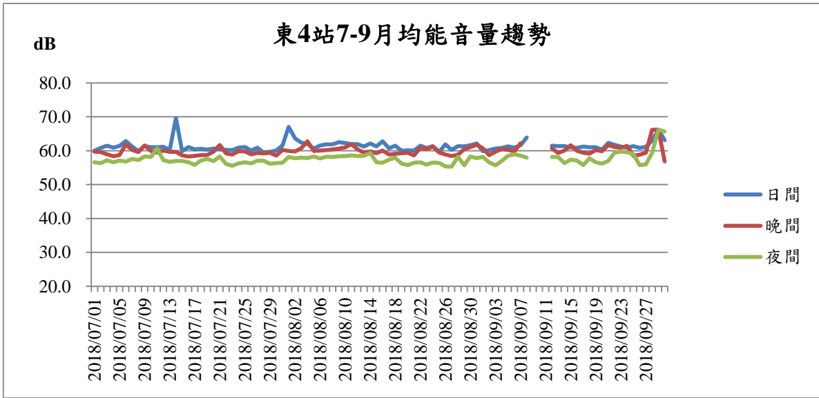
圖8 基隆港東四站107年7-9月噪音監測結果趨勢圖
