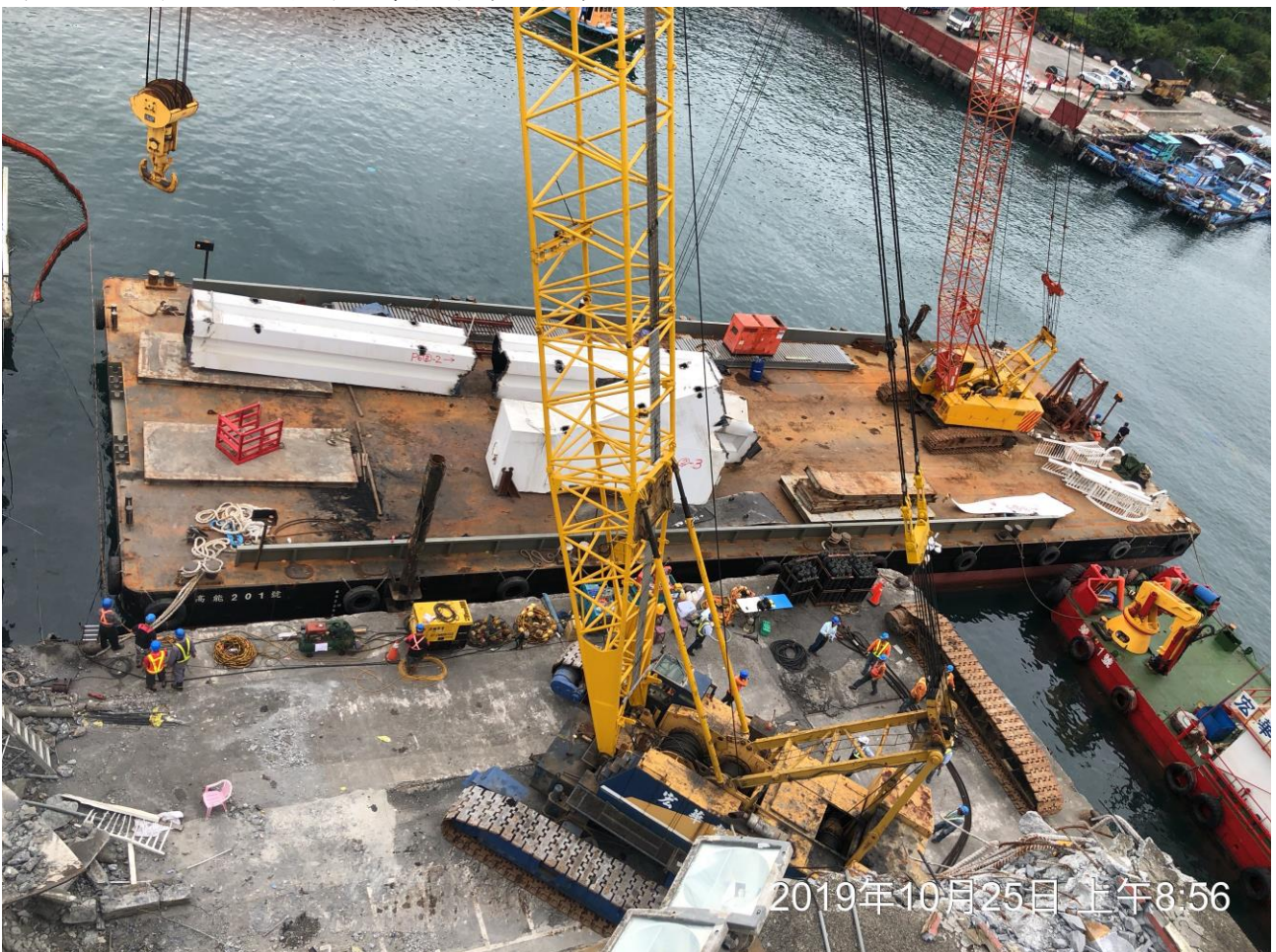
圖 2. 移山陸側 Y 型鋼樑以新加入之高能 201 號平台船吊離情況
