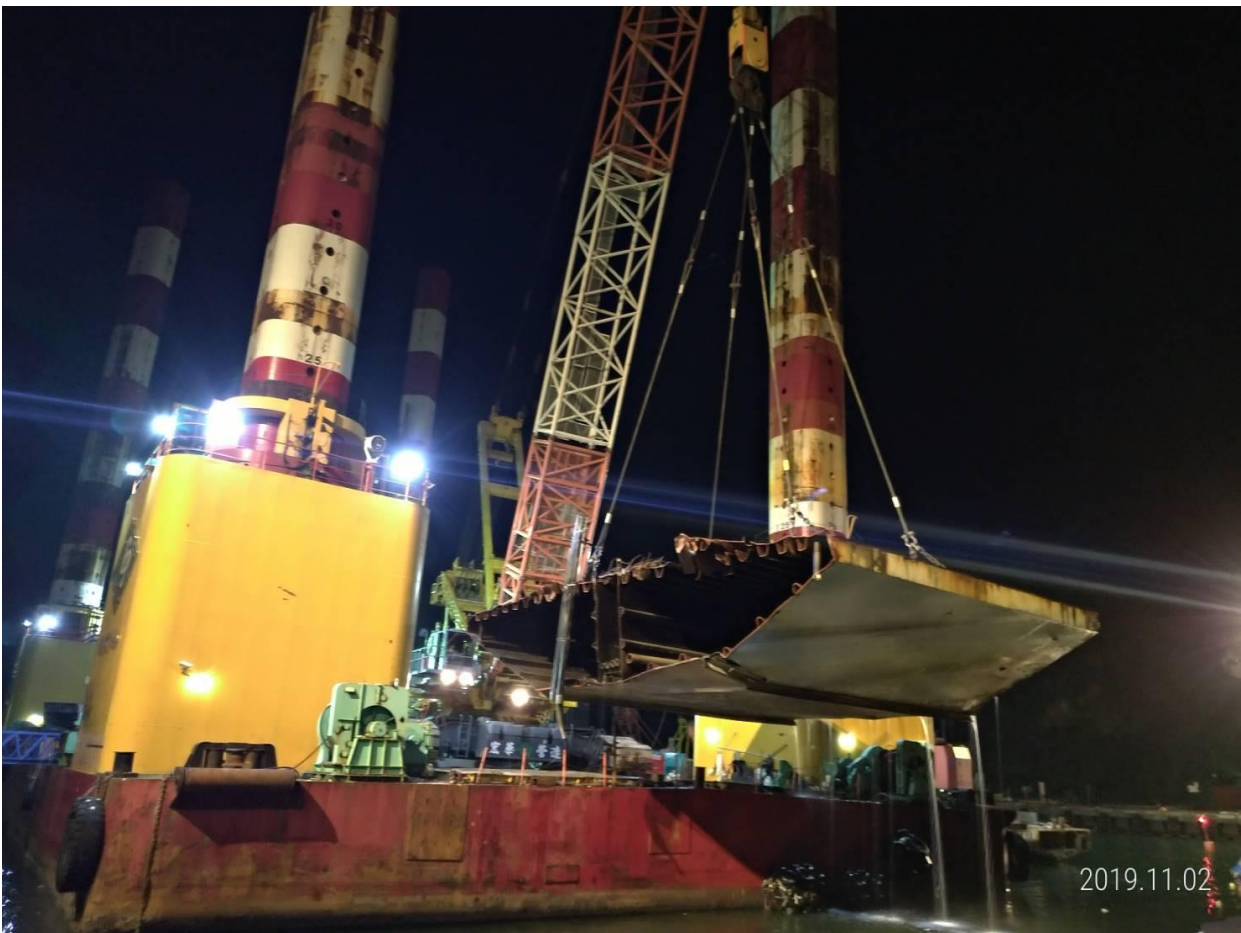
圖 1：宏禹 1 號今吊起移山路側橋面版情況
