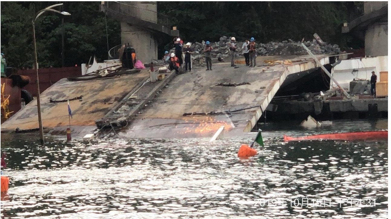
圖 2: 進行橋面版切割準備作業
