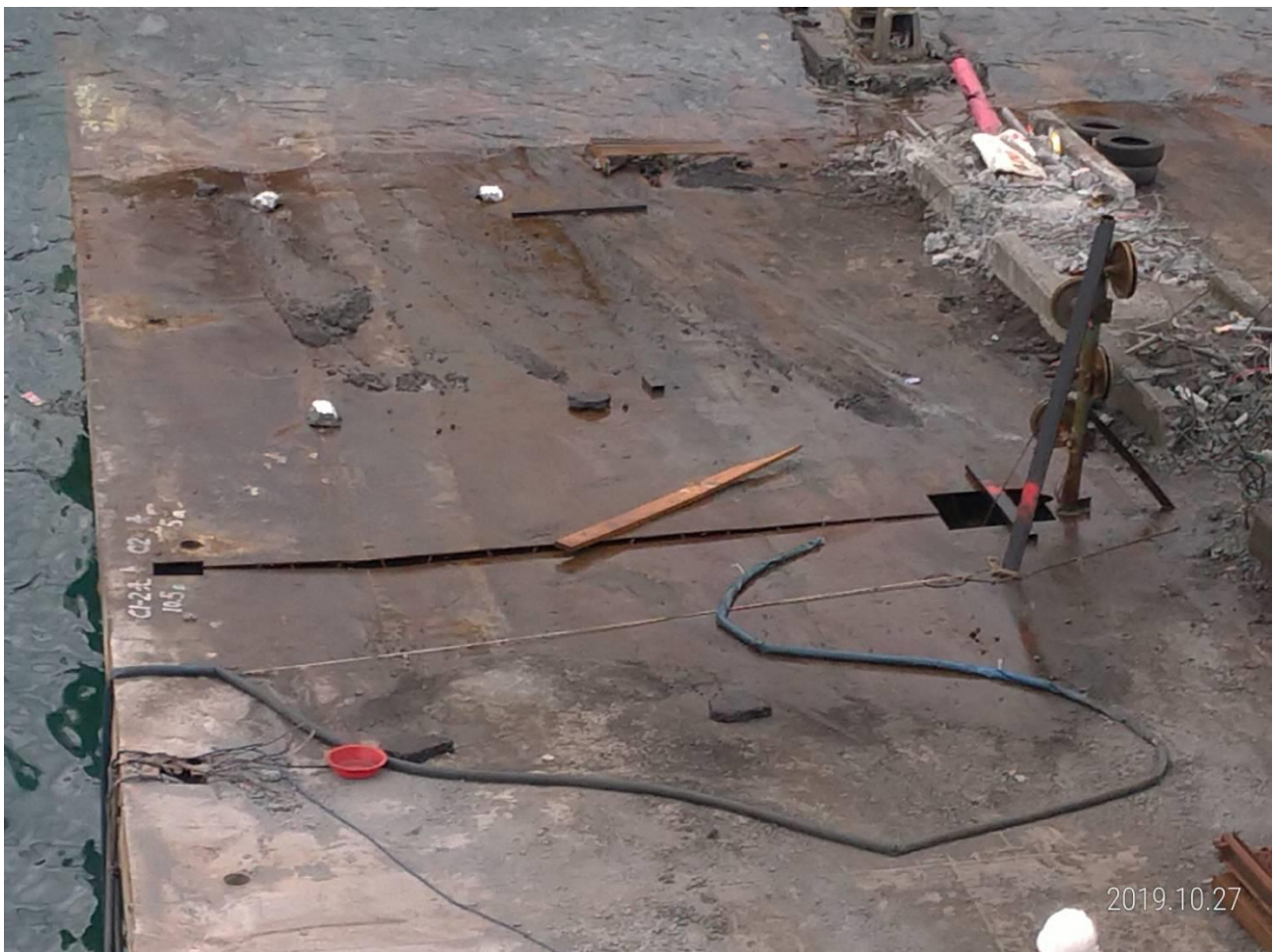
圖 1 南方澳跨海大橋移山路側橋面版第二條切割線處理情形
