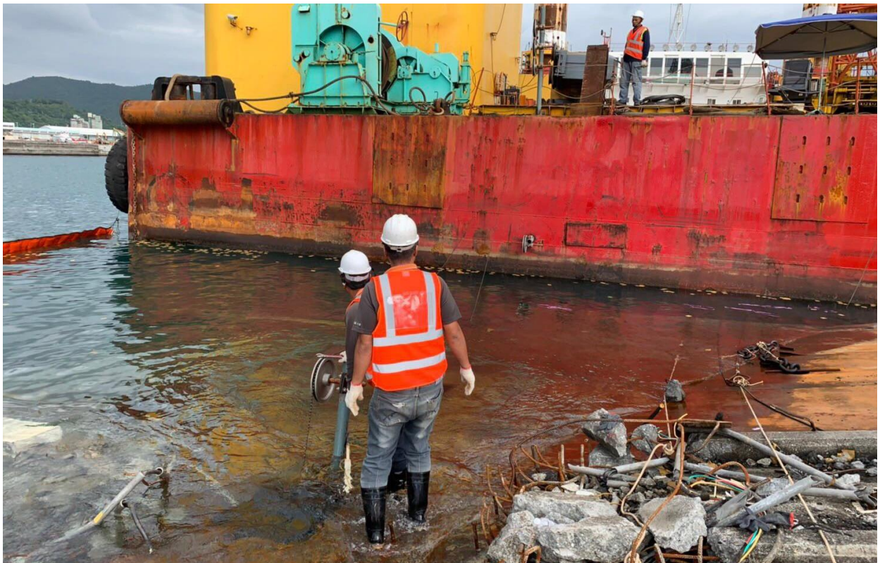
圖 1：鑽石鏈鋸切割橋面版施工狀況
