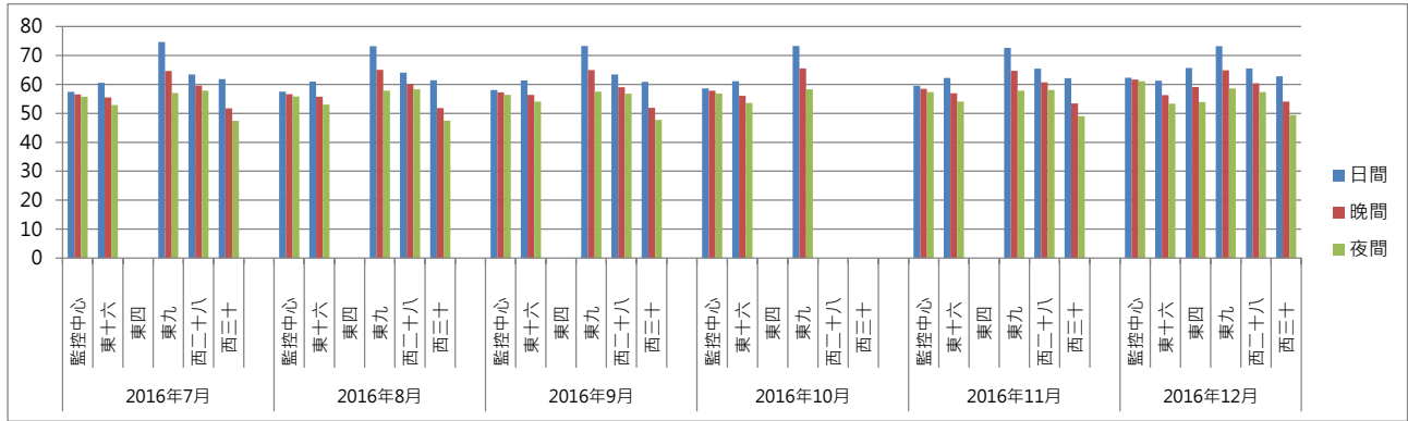
圖6 基隆港105年7-12月噪音監測結果趨勢圖
