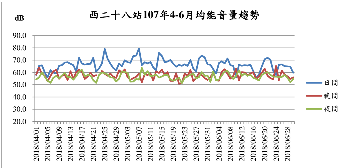
圖10 基隆港西二十八站107年4-6月噪音監測結果趨勢圖
