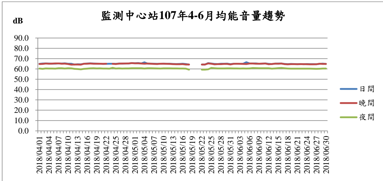
圖6 基隆港監測中心站107年4-6月噪音監測結果趨勢圖
