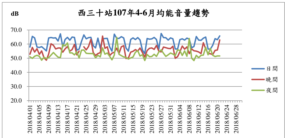
圖11 基隆港西三十站107年4-6月噪音監測結果趨勢圖
