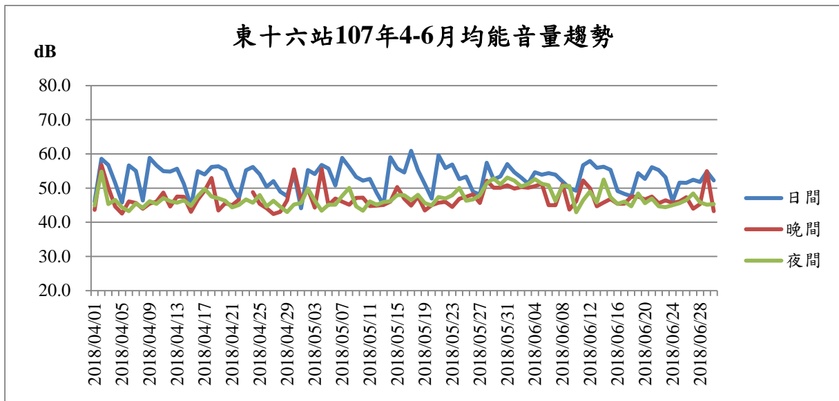
圖7 基隆港東十六站107年4-6月噪音監測結果趨勢圖
