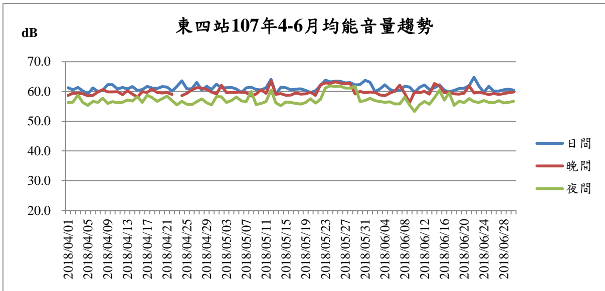
圖8 基隆港東四站107年4-6月噪音監測結果趨勢圖
