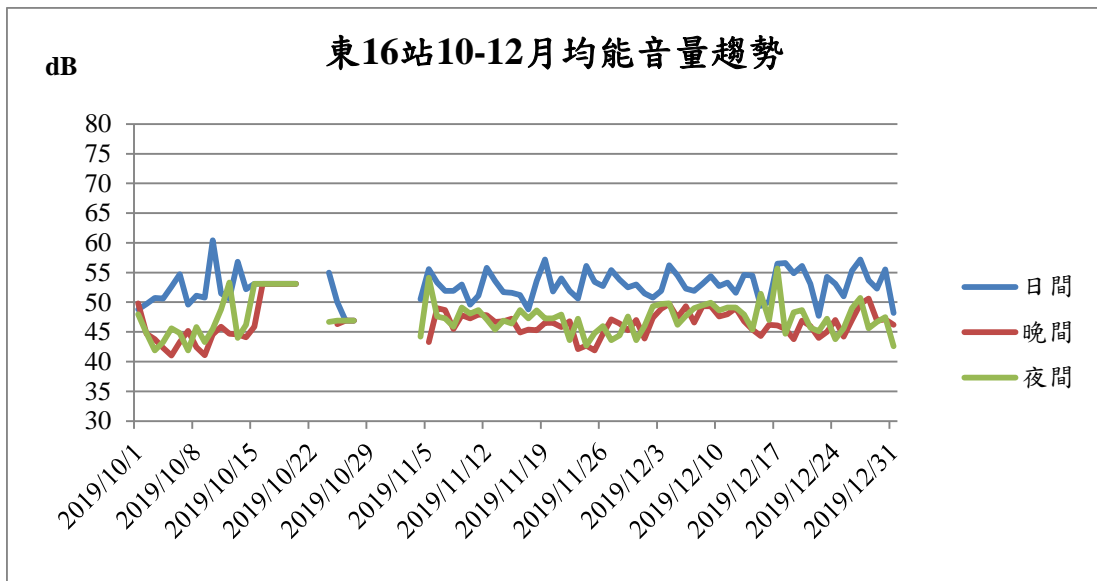
圖7 基隆港東十六站108年10-12月噪音監測結果趨勢圖
