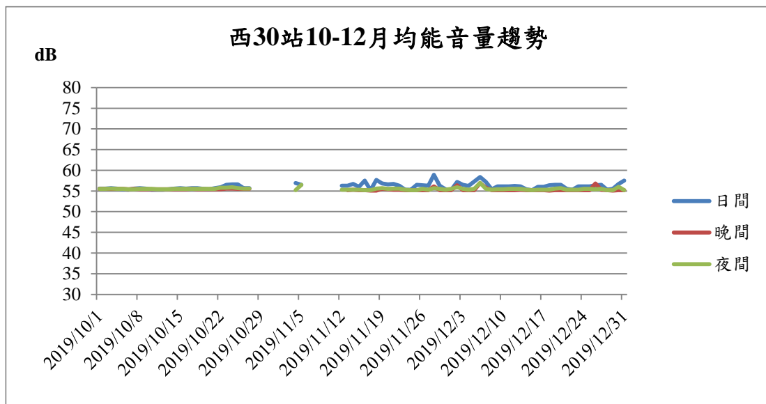
圖11 基隆港西三十站108年10-12月噪音監測結果趨勢圖
