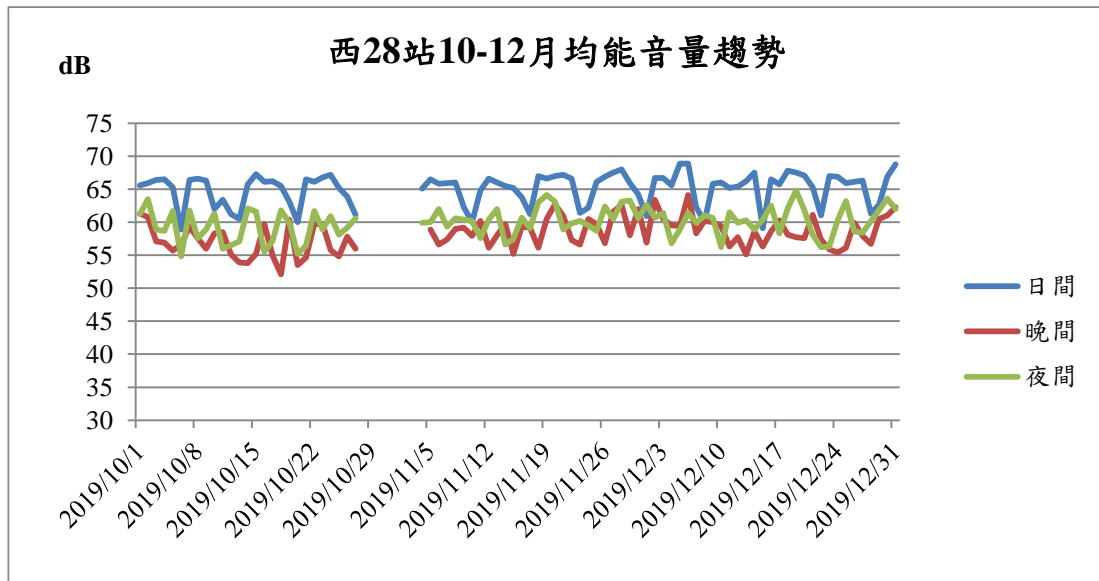
圖10 基隆港西二十八站108年10-12月噪音監測結果趨勢圖
