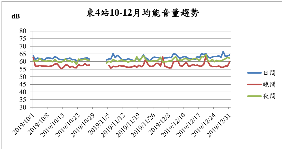
圖8 基隆港東四站108年10-12月噪音監測結果趨勢圖
