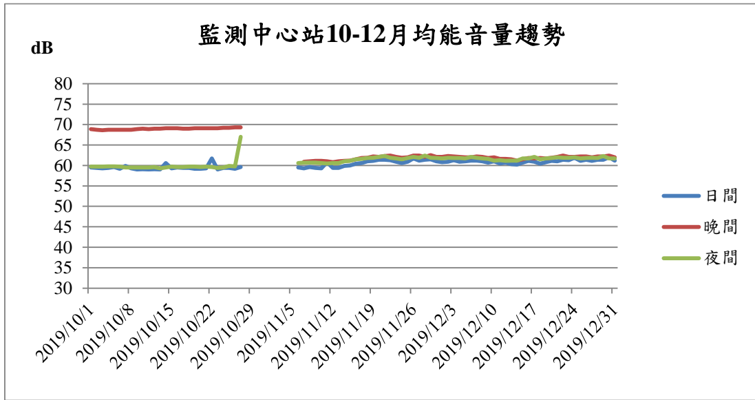
圖6 基隆港監測中心站108年10-12月噪音監測結果趨勢圖
