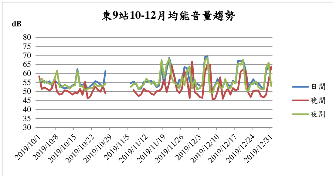
圖9 基隆港東九站108年10-12月噪音監測結果趨勢圖
