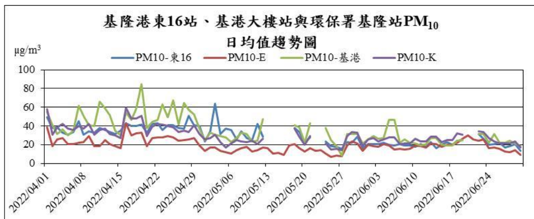
圖1 基隆港東十六站、基港大樓站、基隆港站與環保署基隆站懸浮微粒日均值趨勢圖
