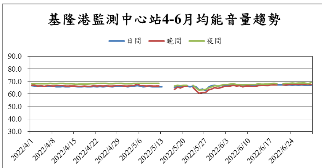
圖6 基隆港監測中心站111年4-6月噪音監測結果趨勢圖
