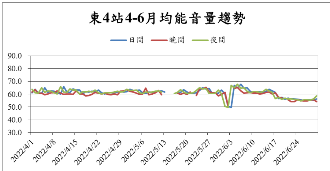
圖8 基隆港東四站111年4-6月噪音監測結果趨勢圖
