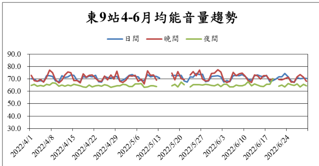
圖9 基隆港東九站111年4-6月噪音監測結果趨勢圖
