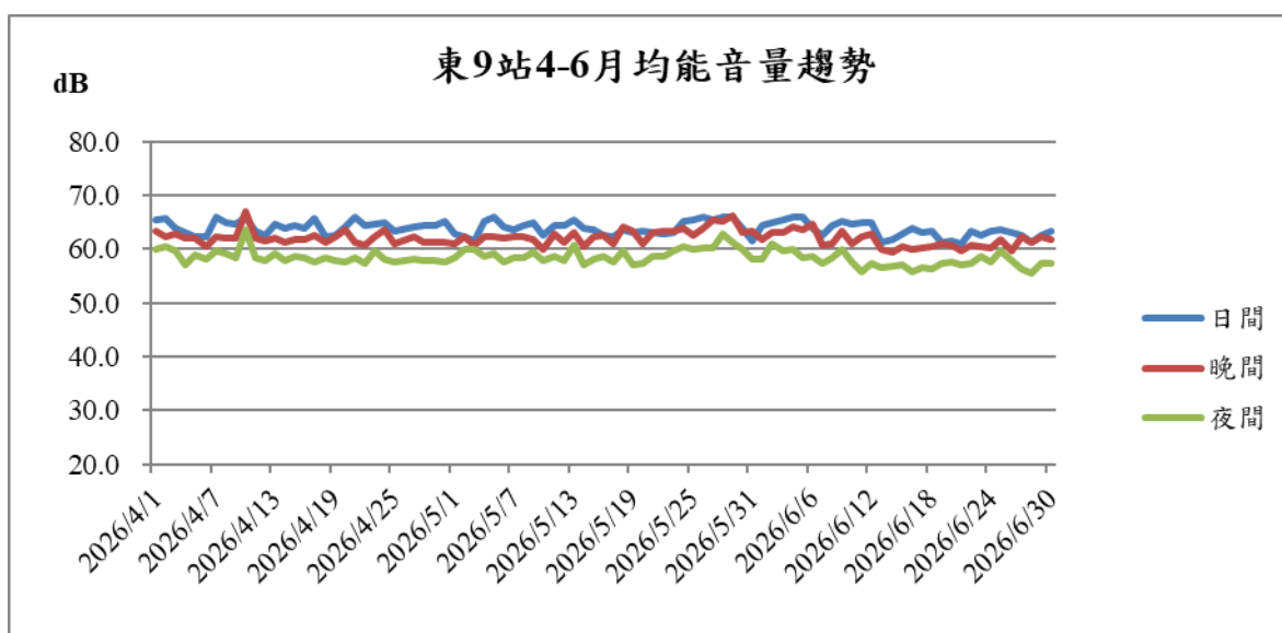
圖9 東九站115年4-6月噪音監測結果趨勢圖
