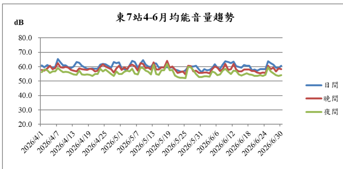
圖8 東七站115年4-6月噪音監測結果趨勢圖
