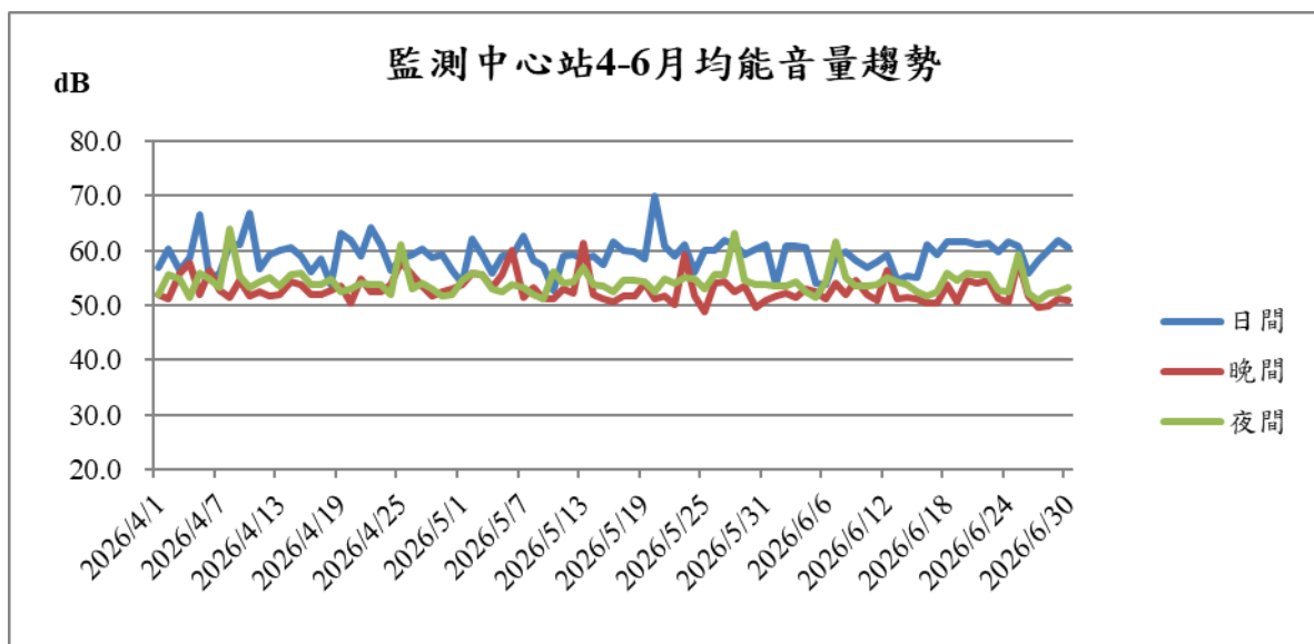
圖6 監測中心站115年4-6月噪音監測結果趨勢圖
