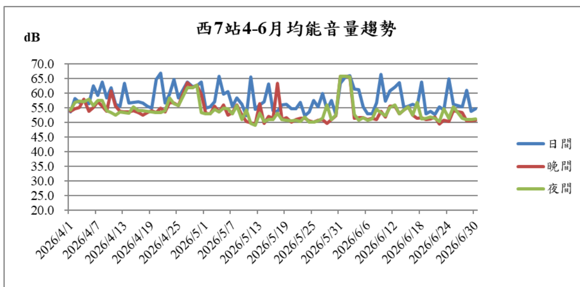
圖10 西七站115年4-6月噪音監測結果趨勢圖
