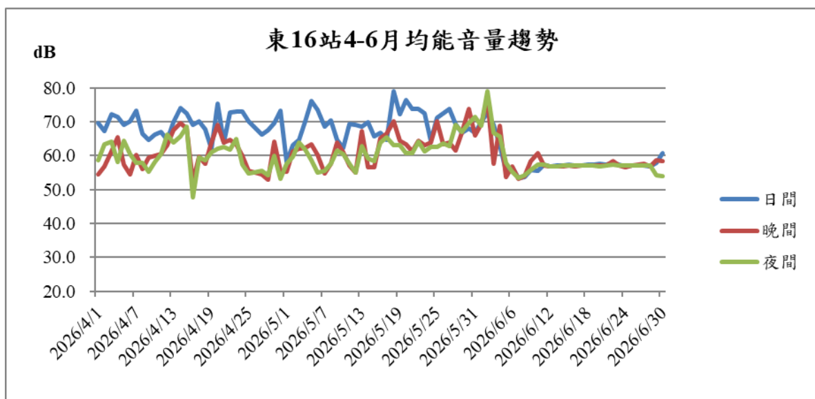
圖7 東十六站115年4-6月噪音監測結果趨勢圖
