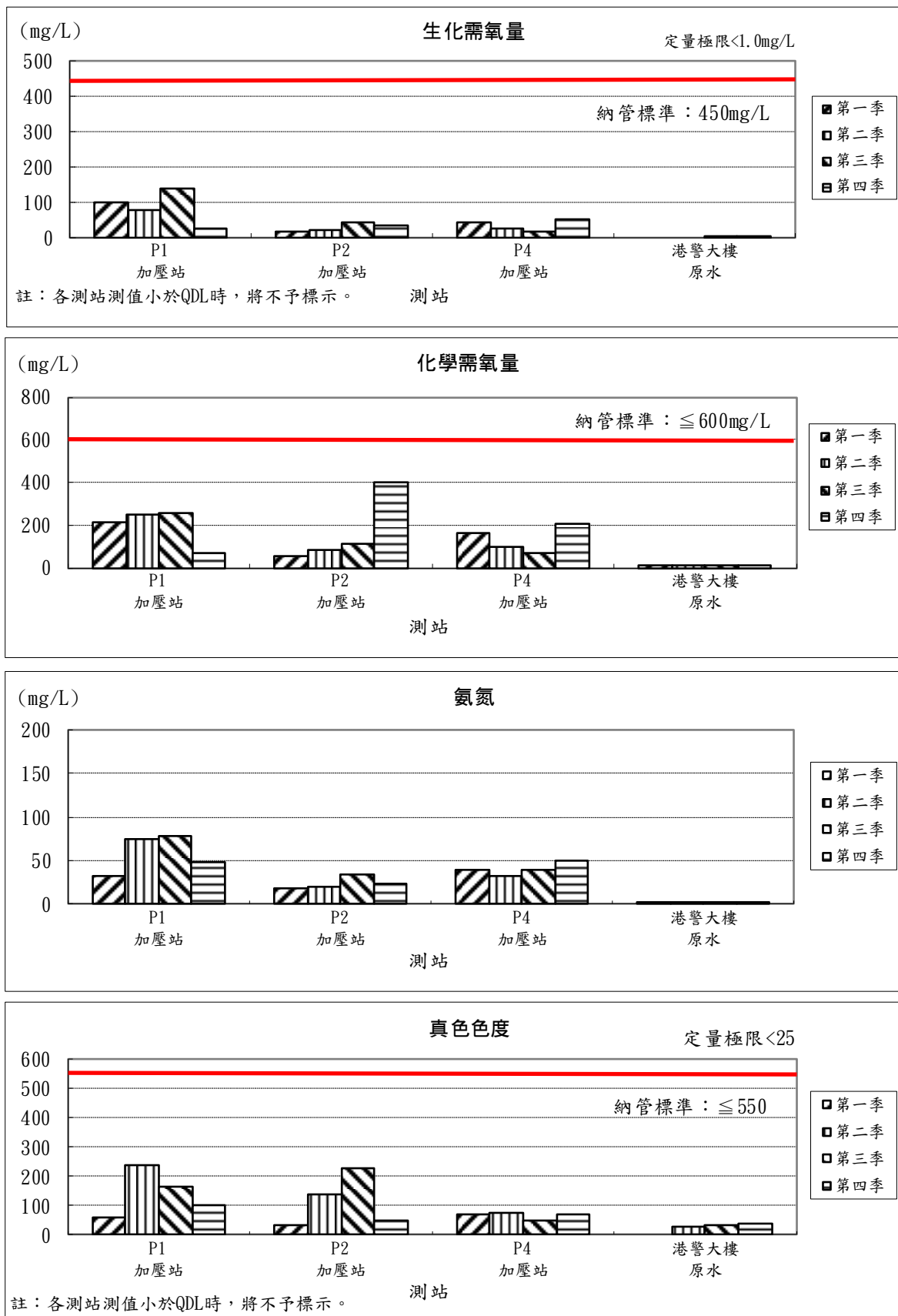
圖 2.1.6-1 本(111)年度港區納管水質監測結果趨勢變化(2/5)
