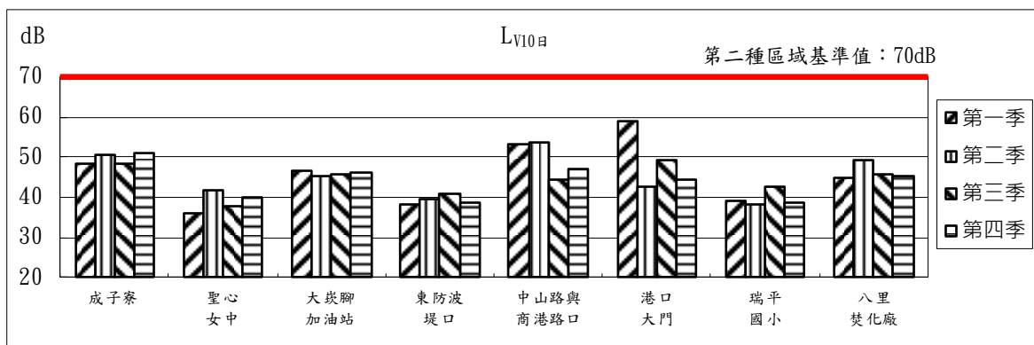
圖 2.1.2-3 本(111)年度假日振動趨勢變化
