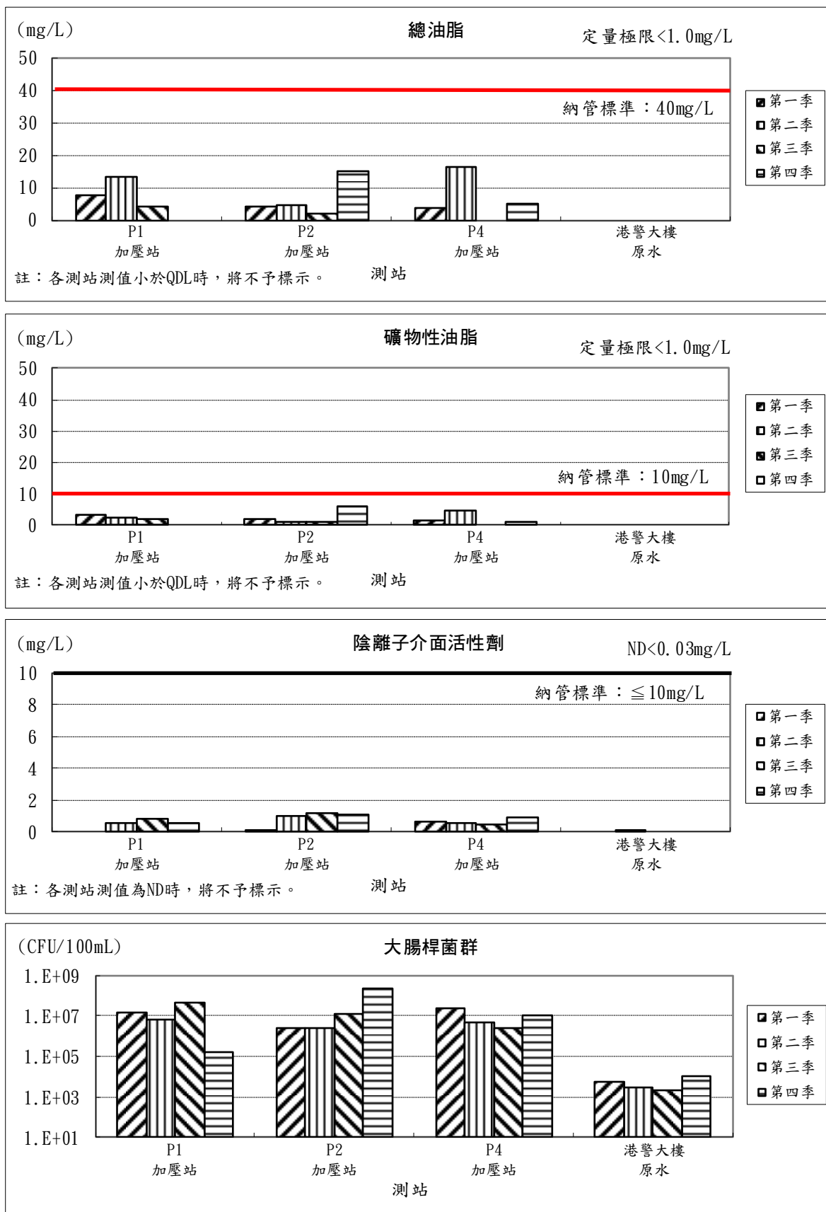
圖 2.1.6-1 本(111)年度港區納管水質監測結果趨勢變化(3/5)
