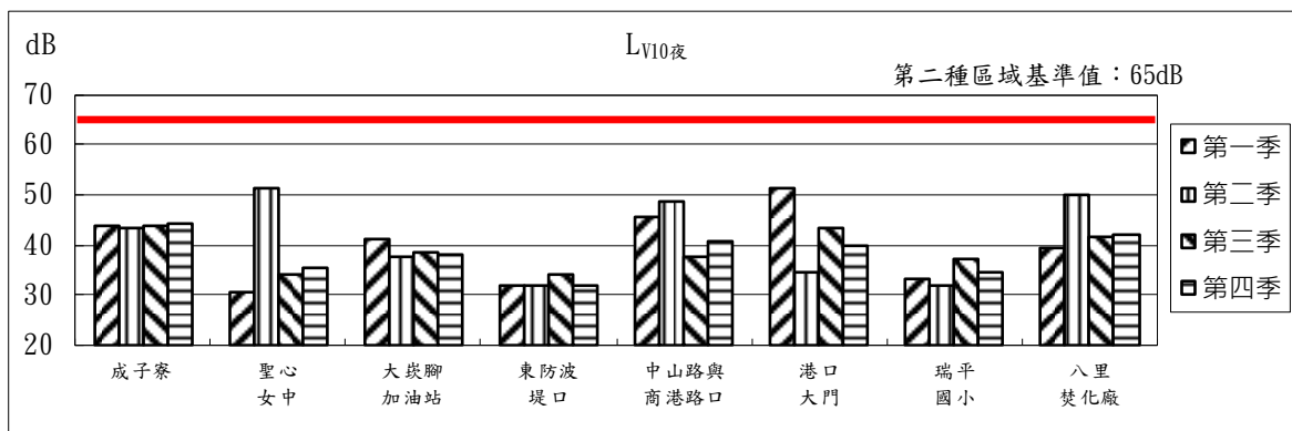
圖 2.1.2-4 本(111)年度非假日振動趨勢變化
