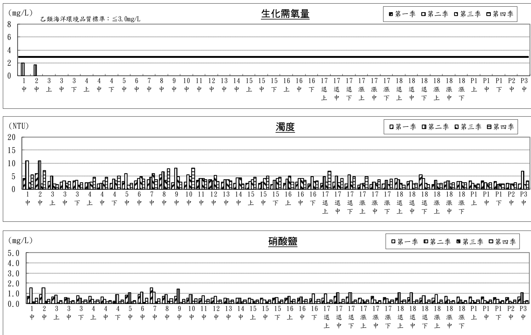
圖 2.1.3-1 本(111)年度海域水質監測結果趨勢變化(5/12)
